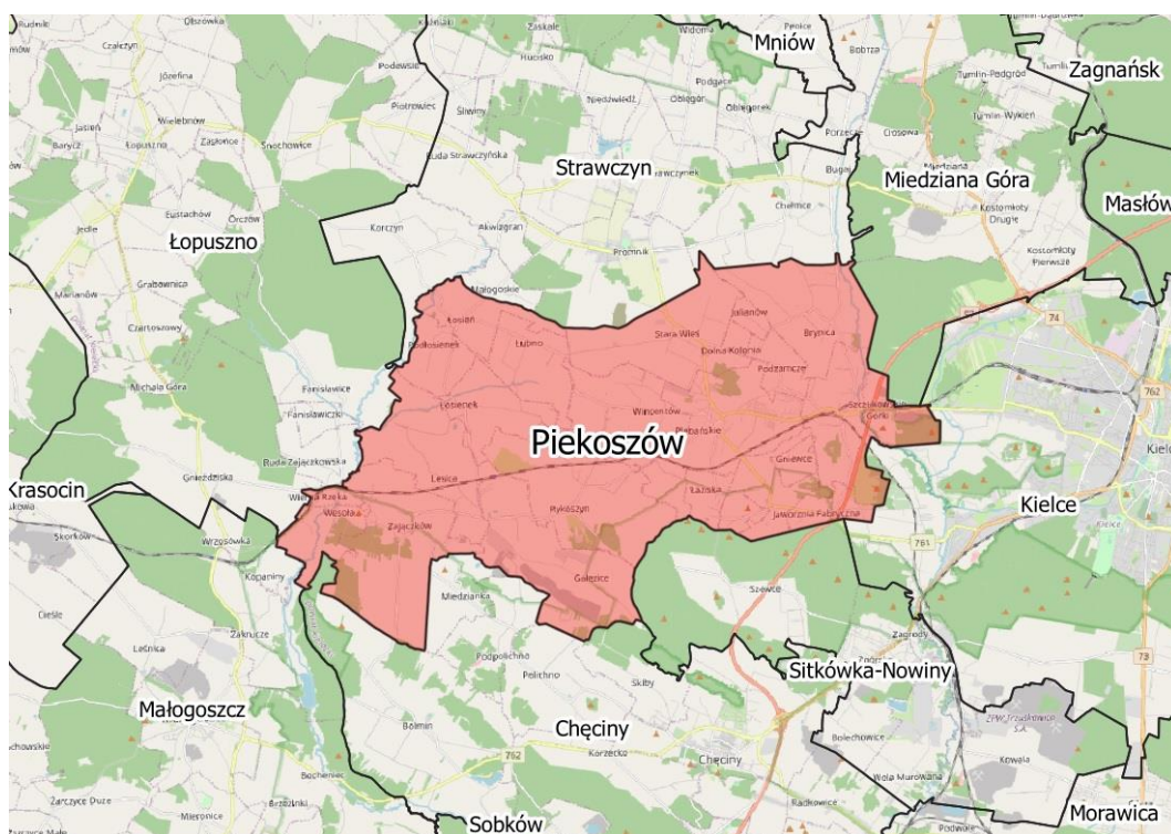
Rysunek 1. Położenie Gminy Piekoszków
