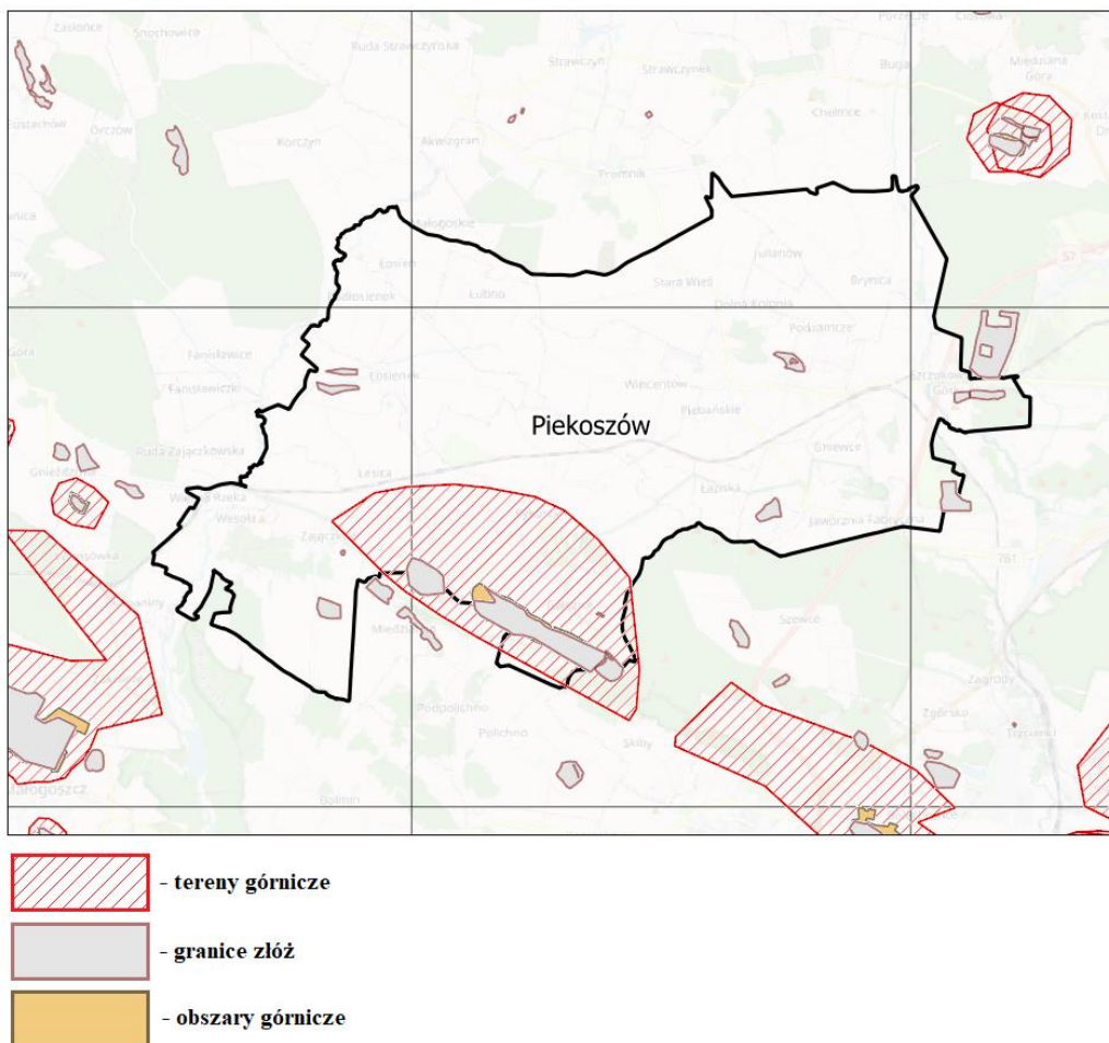
Rysunek 9. Złóża na terenie Gminy Piekoszów
