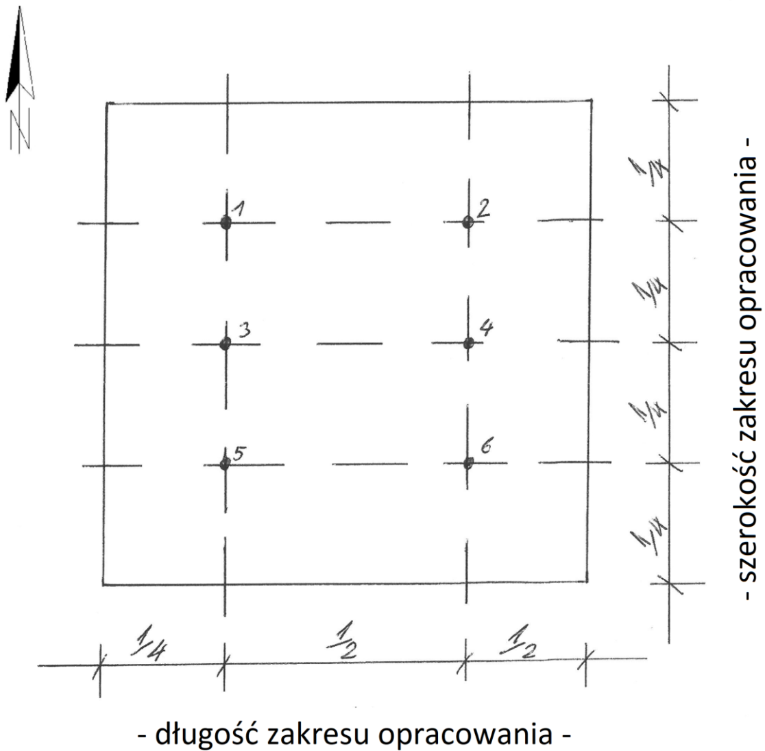
Schemat – umiejscowienie otworów badawczych geotechnicznych – 6 szt.
